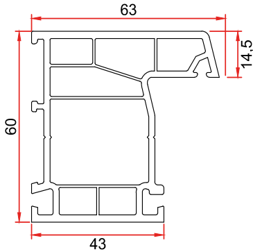
Mamül Kodu/Product Code/Код изделия: 4044 L Kasa 43mm L Frame 43mm Рама L 43мм
