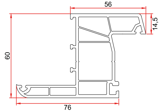
Mamül Kodu/Product Code/Код изделия: 4043 Pervazlı L Kasa L Frame with Cornice Рама L с наличником
