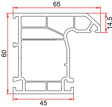
Mamül Kodu/Product Code/Код изделия: 2044 L Kasa L Frame Рама L
