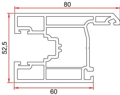
Mamül Kodu/Product Code/Код изделия: 3048 Sürme Kanat Sliding Sash Створка раздвижная
