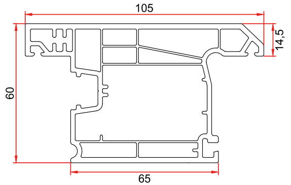
Mamül Kodu/Product Code/Код изделия: 2021 Dışa Açılır T Kapı Kanat Outside Opening T Door Sash Дверная створка T наружного открывания
