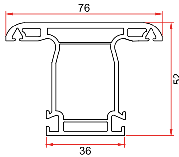
Mamül Kodu/Product Code/Код изделия: 3052 Sürme T Orta Kayıt Sliding T Mullion Импост раздвижной T
