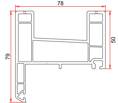
Mamül Kodu/Product Code/Код изделия: 3043 Çift Raylı Pervazlı Sürme Kasa Double Railed Sliding Frame with Cornice Рама раздвижная двойная с наличником
