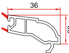
Mamül Kodu/Product Code/Код изделия: 2051 T Orta Kayıt T Mullion Импост T
