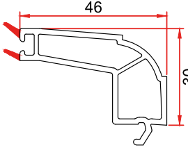
Mamül Kodu/Product Code/Код изделия: 7040 Kasa Tek Cam Çıtası Frame Single Glazing Bead Штапик рамы одинарного остекления
