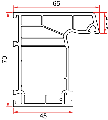
Mamül Kodu/Product Code/Код изделия: 5044 L Kasa L Frame Рама L
