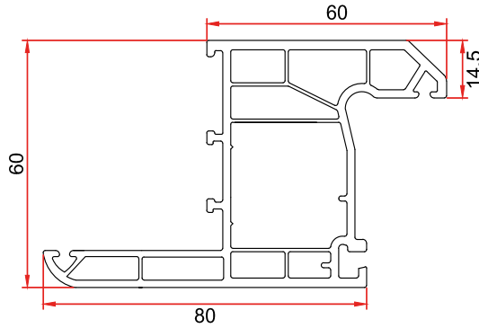
Mamül Kodu/Product Code/Код изделия: 2043 Pervazlı L Kasa L Frame with Cornice Рама L с наличником
