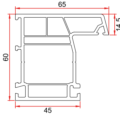
Mamül Kodu/Product Code/Код изделия: 4045 L Kasa 45mm L Frame 45mm Рама L 45мм
