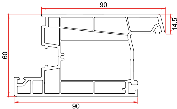
Mamül Kodu/Product Code/Код изделия: 4060 Z Kapı Kanat Z Door Sash Дверная створка Z
