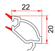
Mamül Kodu/Product Code/Код изделия: 7036 4x16x4 Çift Cam Çıtası 4x16x4 Double Glazing Bead Штапик двойного остекления 4x16x4
