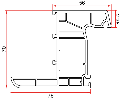
Mamül Kodu/Product Code/Код изделия: 5043 Pervazlı L Kasa L Frame with Cornice Рама L с наличником
