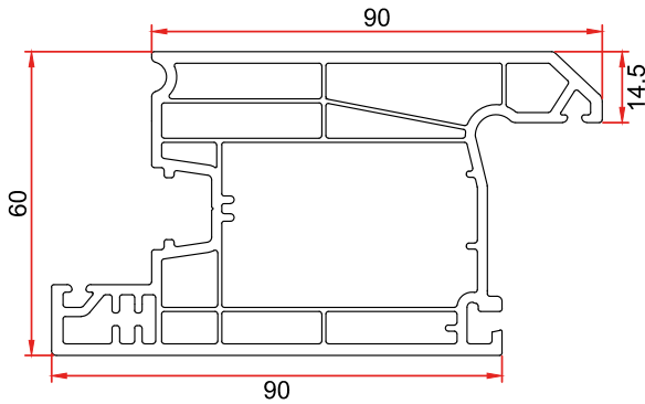
Mamül Kodu/Product Code/Код изделия: 2060 Z Kapı Kanat Z Door Sash Дверная створка Z
