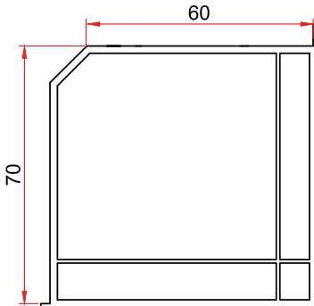
Mamül Kodu/Product Code/Код изделия: Y010 60/70mm Kutu Profili 60/70mm Box Profile Профиль коробки 60/70мм
