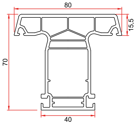
Mamül Kodu/Product Code/Код изделия: 5051 T Orta Kayıt T Mullion Импост T
