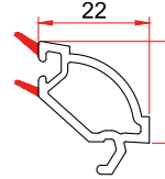
Mamül Kodu/Product Code/Код изделия: 7036 Kanat 4x16x4 Çift Cam Çıtası Sash 4x16x4 Double Glazing Bead Штапик створки двойного остекления 4X16X4
