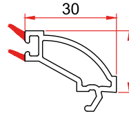
Mamül Kodu/Product Code/Код изделия: 7035 Kanat 4x12x4 Çift Cam Çıtası Sash 4x12x4 Double Glazing Bead Штапик створки двойного остекления 4x12x4
