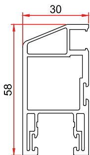
Mamül Kodu/Product Code/Код изделия: 3082 Sürme Sineklik Kanat Sliding Flynet Sash Москитная раздвижная створка
