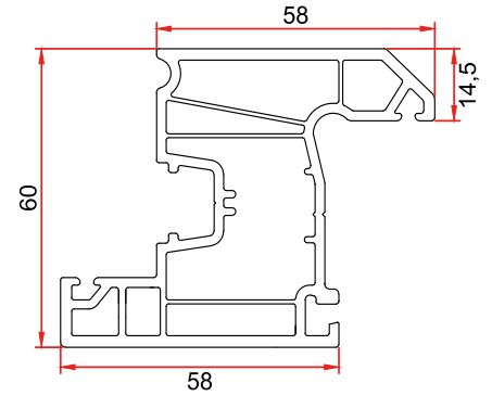
Mamül Kodu/Product Code/Код изделия: 2034 Z Pencere Kanat Z Window Sash Оконная створка Z
