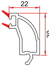
Mamül Kodu/Product Code/Код изделия: 7039 Kasa 4x16x4 Çift Cam Çıtası Frame 4x16x4 Double Glazing Bead Штапик рамы двойного остекления 4X16X4
