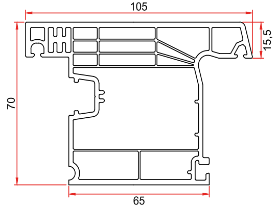
Mamül Kodu/Product Code/Код изделия: 5021 Dışa Açılır T Kapı Kanat Outside Opening T Door Sash Дверная створка T наружного открывания
