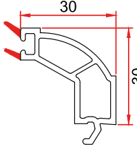
Mamül Kodu/Product Code/Код изделия: 7041 Kasa 4x12x4 Çift Cam Çıtası Frame 4x12x4 Double Glazing Bead Штапик рамы двойного остекления 4x12x4
