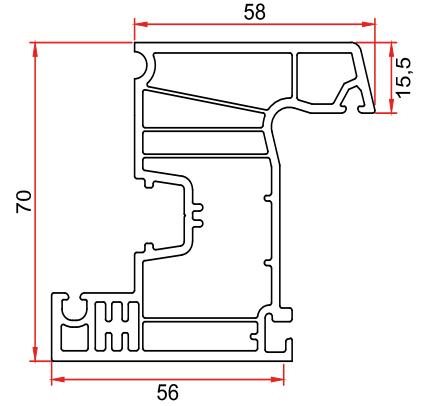
Mamül Kodu/Product Code/Код изделия: 5034 Z Pencere Kanat Z Window Sash Оконная створка Z
