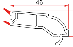
Mamül Kodu/Product Code/Код изделия: 7040 Kasa Tek Cam Çıtası Frame Single Glazing Bead Штапик рамы одинарного остекления
